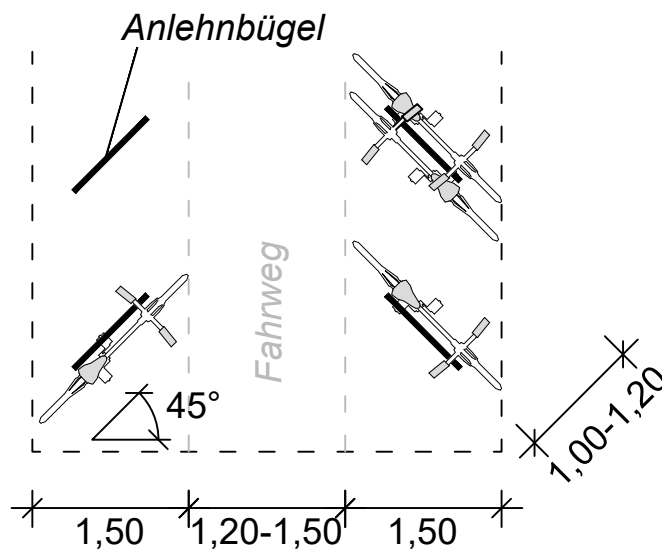
Schrägaufstellung mit Anlehnbügel
