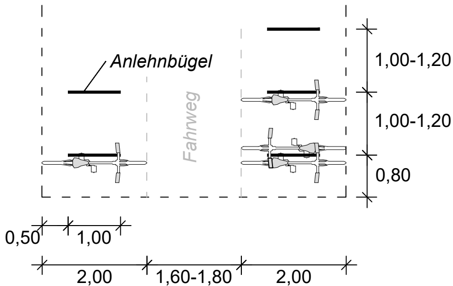
Queraufstellung mit Anlehnbügel
